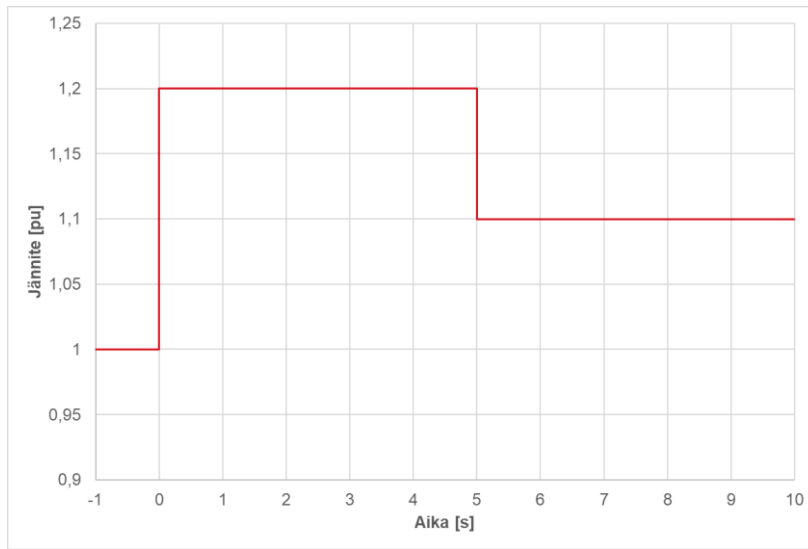
Kuva 10.4. Lyhytaikaista ylijännitettä vastaava liittymispisteen pääjännite, jonka aikana ja jälkeen tyypin B, C ja D voimalaitosten tulee jatkaa toimintaansa normaalisti. Jännitteen suhteellisarvo 1,0 pu on liittymispisteen normaali käyttö-jännite ennen häiriötä.
