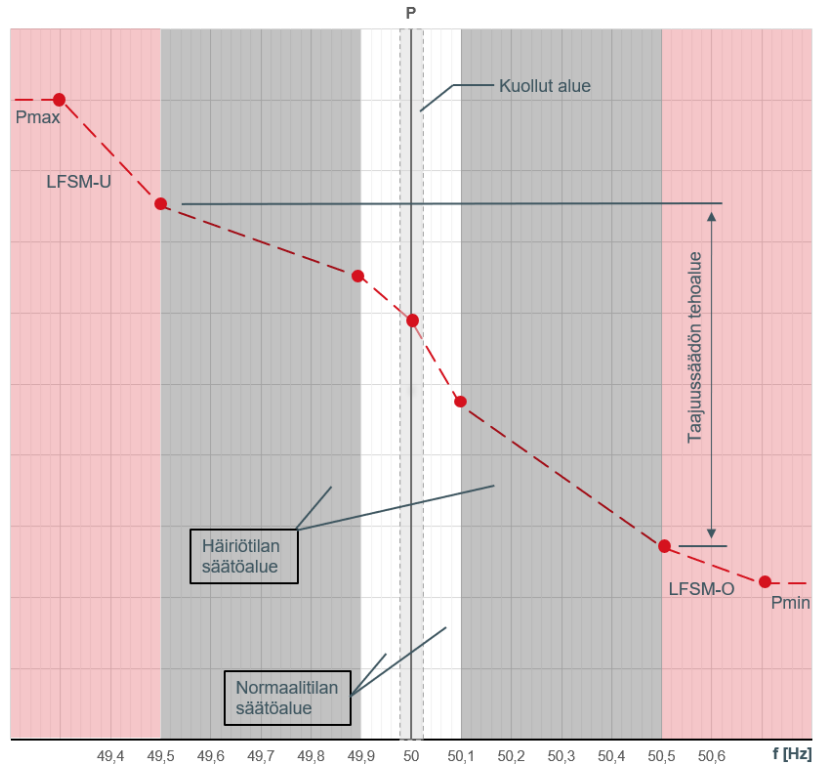
Kuva 16.1. Tajuuussäädön jatkuva toiminta eri taajuusalueilla. Kaikille taajuusalueille on omat statiikka- ja tehoraja-asettelunsa. Kuollut alue 50 Hz:n ympärillä on aseteltavissa erikseen. Kuvassa esitetyt taajuusarvot, statiikka-asettelut ja tehoalueet ovat esimerkinomaisia. Tehotasot P_{max} ja P_{min} kuvaavat suurinta ja pienintä säätötasoa.
