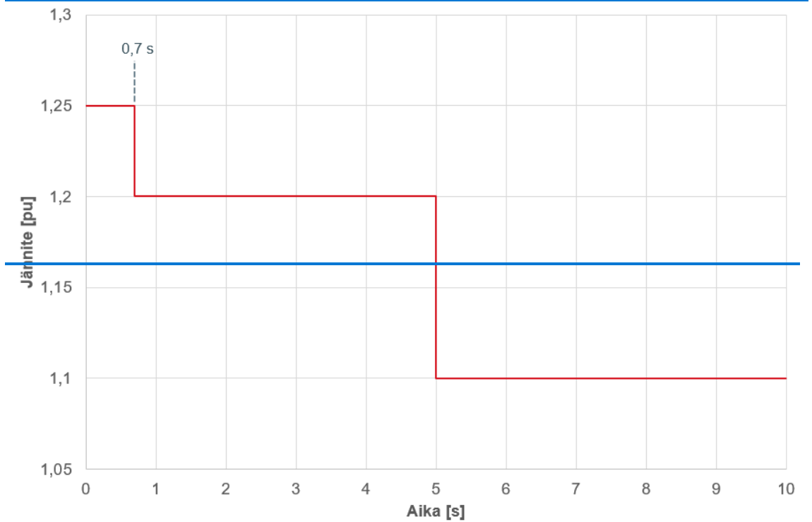
Kuva 10.2. Lyhytaikaista ylijännitettä vastaava liittämispisteen pääjännite, jonka aikana ja jälkeen tyyppin B, C ja D sähkövarastojen tulee jatkaa toimintaansa normaalisti. Jännitteen suhteellisarvo 1,0 pu on liittämispisteen normaali käyttöjännite ennen häiriötä.
