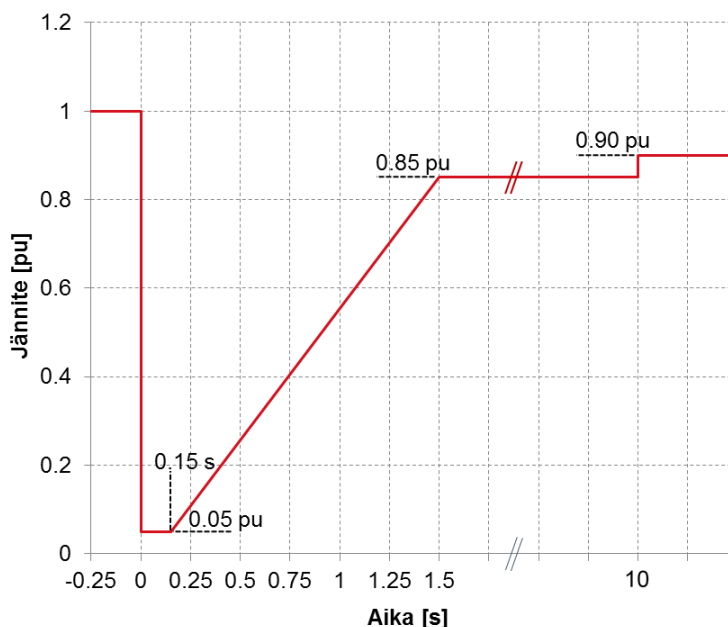
Kuva 10.1. Lyhytaikaista jännitehäiriötä vastaava liittymispisteen jännite, jonka aikana ja jälkeen tyyppiin B ja C sähkövarastojen tulee jatkaa toimintaansa normaalisti. Jännitteen suhteellisarvo 1,0 pu on jännite ennen häiriötä. Jännite on 0,05 pu 150 millisekunnin ajan.
