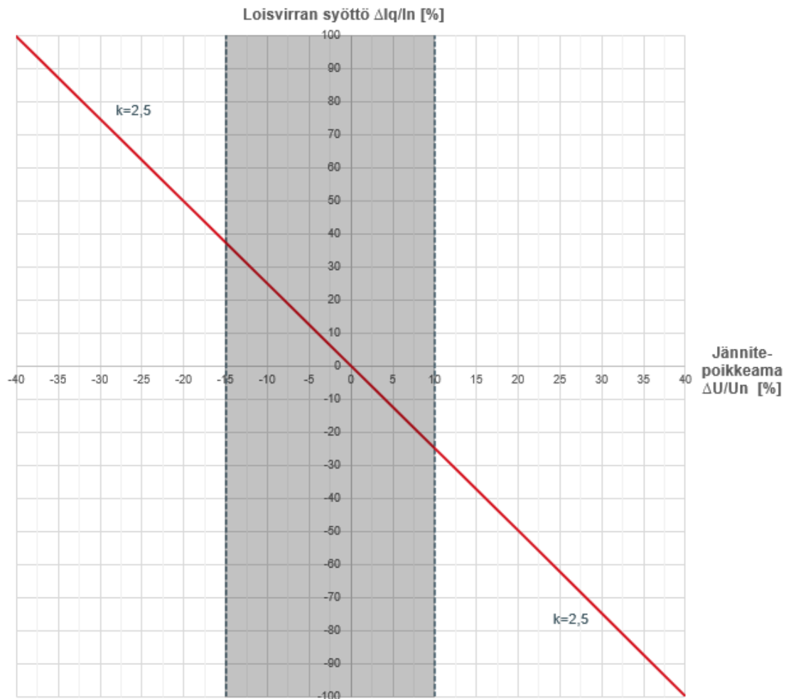
Kuva 10.3. Loisivirran aktivointirajat jännitteen perusteella sekä k-kertoimen määrittely. Loisivirran syöttö aktivoituu harmaaan alueen ulkopuolella. Suora kuvaa kulmakertoa k=2,5 .
