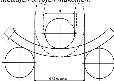
Taivutuskokeen kaaviokuva
