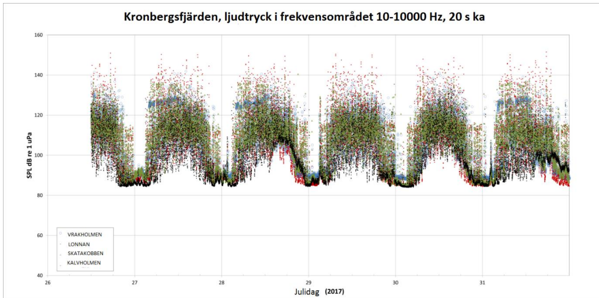
Bild 21. Bullermätning i Kronobergsfjärden med bottenförankrade hydrofonloggers i juli 2017. Preliminära resultat. Ljudtryck för bredbandsbuller vid fyra mätpunkter: Vrakholmen, Lonna, Skata, Kalvholmen. Årstidsvariationerna är tydliga vid alla mätpunkter. De tystaste timmarna är dygnets två första timmar. Ljudnivån är förvånansvärt hög vid tre mätpunkter. 140 dB buller i vattnet motsvarar cirka 80 dB buller i luften.
