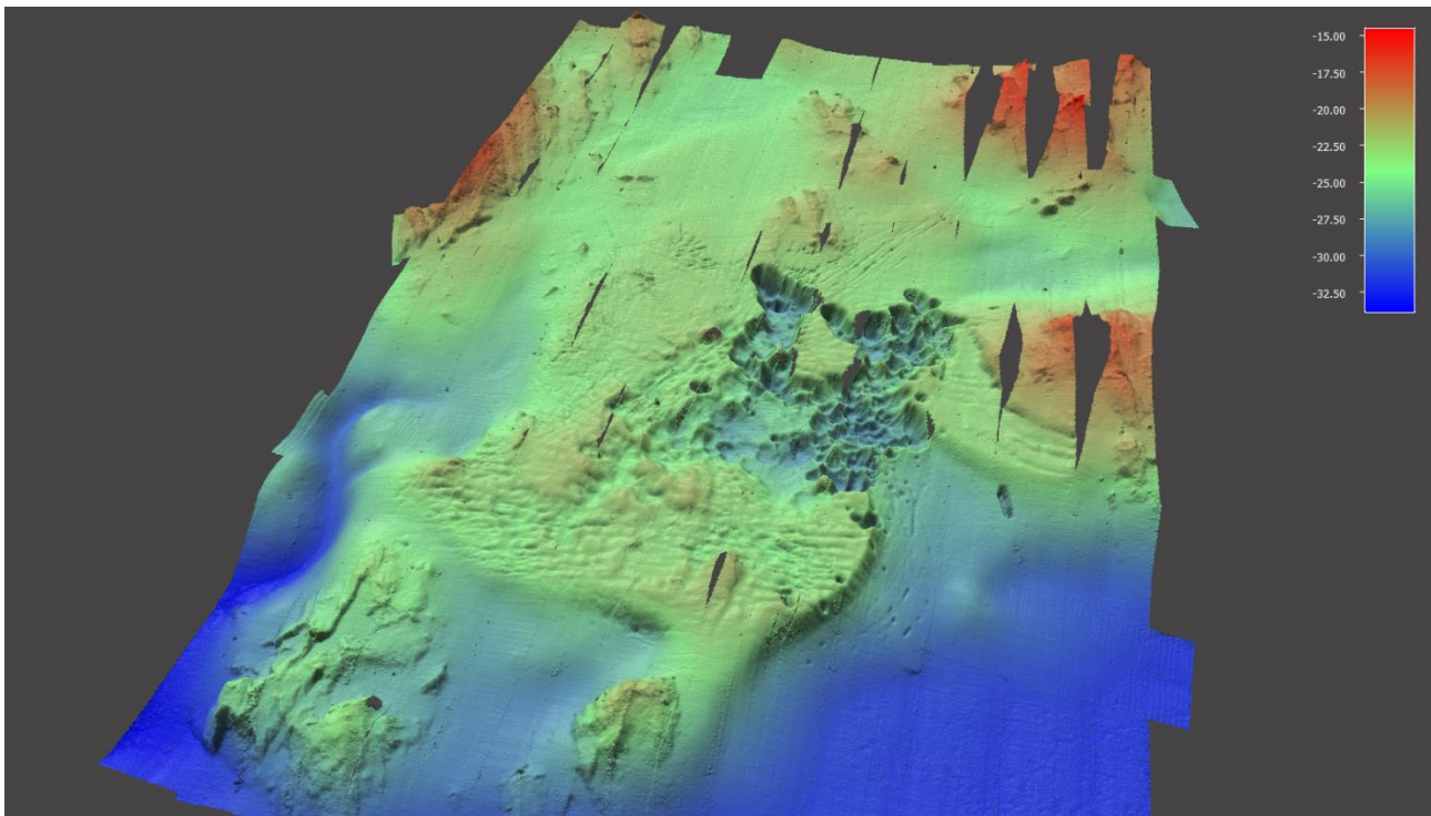
Bild 23. Bottenytans form vid en havssandtäkt i området runt Estlotan utanför Helsingfors. Foto från multibeammätning år 2015 som visar spår och rundgrovar efter muddring (GTK).
