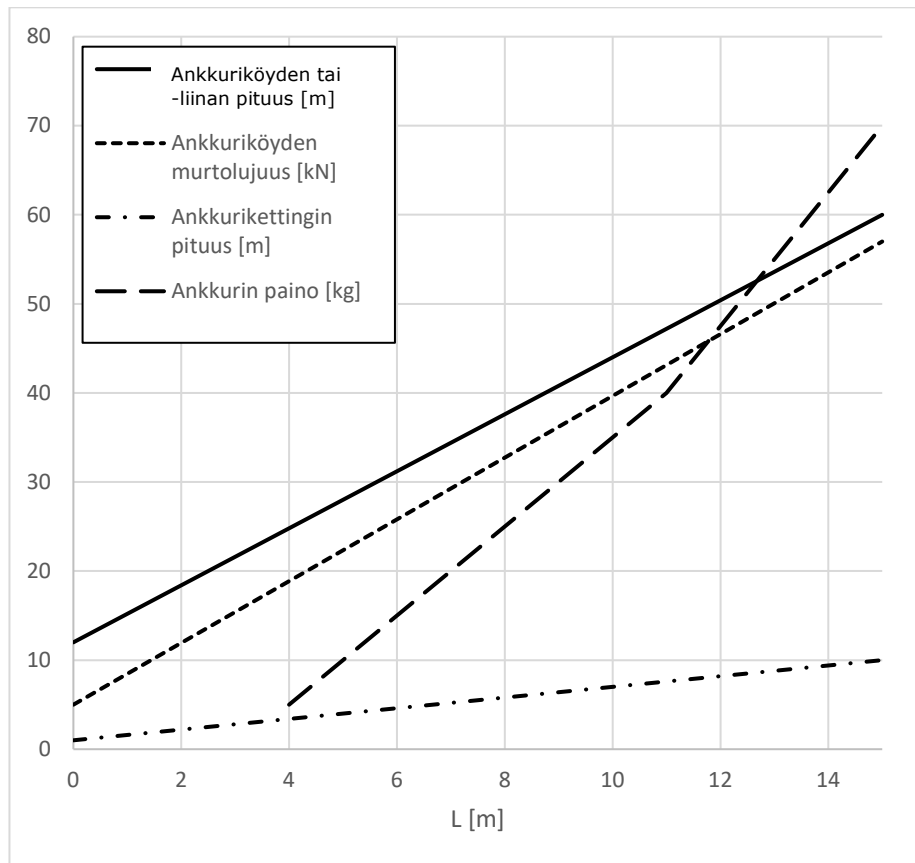
Kuva 1 Alle 15 metrin pituisen perinnealuksen ankkurivarustuksen mitoitus.
