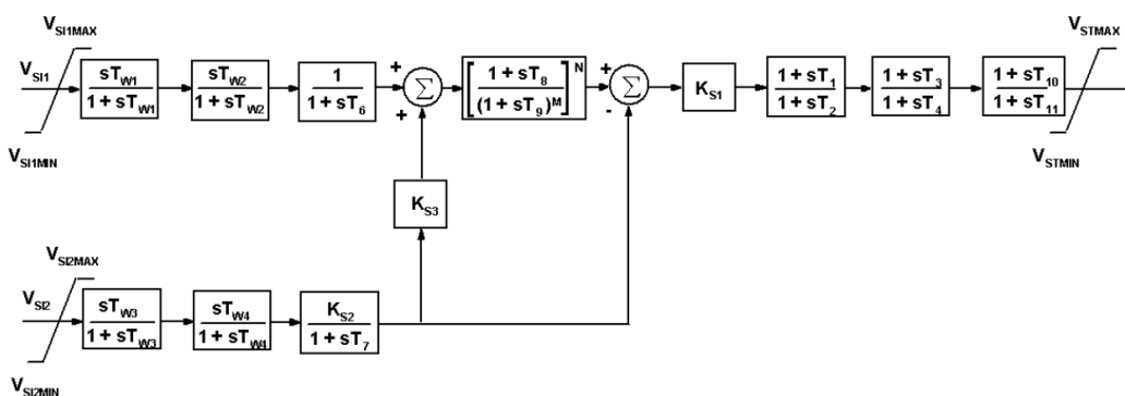
Kuva 22.1. PSS2B lisästabiloinnin lohkokaaviokuva (standardista IEEE 421.5).
