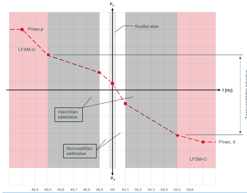
Kuva 11,24. Taajuussäätö. Taajuussäätö toiminnan on oltava jatkuvaa siirtymässä taajuusalueelta toiselle sekä tuotanto- ja kulutustilan välillä. Kaikille taajuusalueille on omat statiikka- ja tehoraja-asettelunsa. Kuollut alue 50 Hz:n ympärillä on aseteltavissa erikseen. Kuvassa esitetyt taajuusarvot, statiikka-asettelut ja tehoalueet ovat esimerkinomaisia. Tehotasot P_{max,p} ja P_{min,d} kuvaavat
