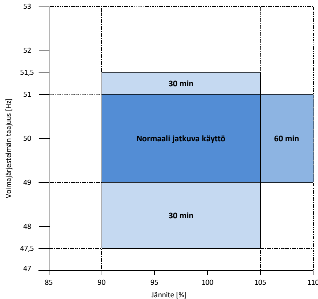
Kuva 10.52. Sähkövaraston on pysyttävä sähköverkkoon kytkeytyneenä kuvassa esitetyillä erilaisilla liittymispisteen taajuuksilla ja jännitteillä. Jatkuvan toiminta-alueen 100 %:n jännite on 400 kV:n verkossa aina 400 kV. Muilla jännitteillä 100 %:n arvoa vastaava jännite on selvitettävä liittymispisteen verkonhaltijalta.
