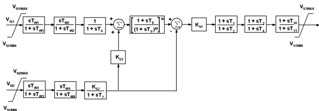
Kuva 22.1. PSS2B lisästabiloinnin lohkokaaaviokuva (standardista IEEE 421.5).
