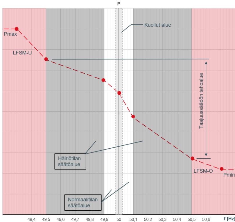
Kuva 16.1. Taajuussäädön jatkuva toiminta eri taajuusalueilla. Kaikille taajuusalueille on omat statiikka- ja tehoraaja-asettelunsa. Kuollut alue 50 Hz:n ympärillä on aseteltavissa erikseen. Kuvassa esitetyt taajuusarvot, statiikka-asettelut ja tehoalueet ovat esimerkinomaisia. Tehotasot P_{max} ja P_{min} kuvaavat suurinta ja pienintä säätötasoa.
